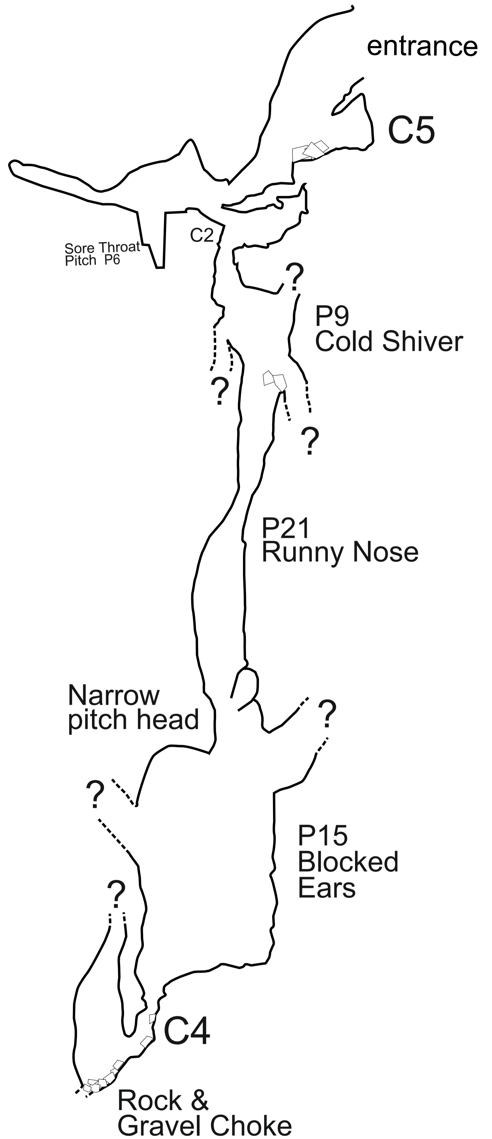
Elevation E-W
